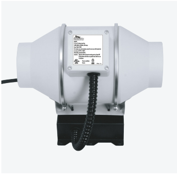
Mixed Flow Fan Assembly
